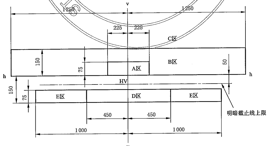
图 1 配光屏幕
